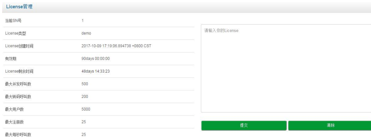
图 3-6-12 License 管理
